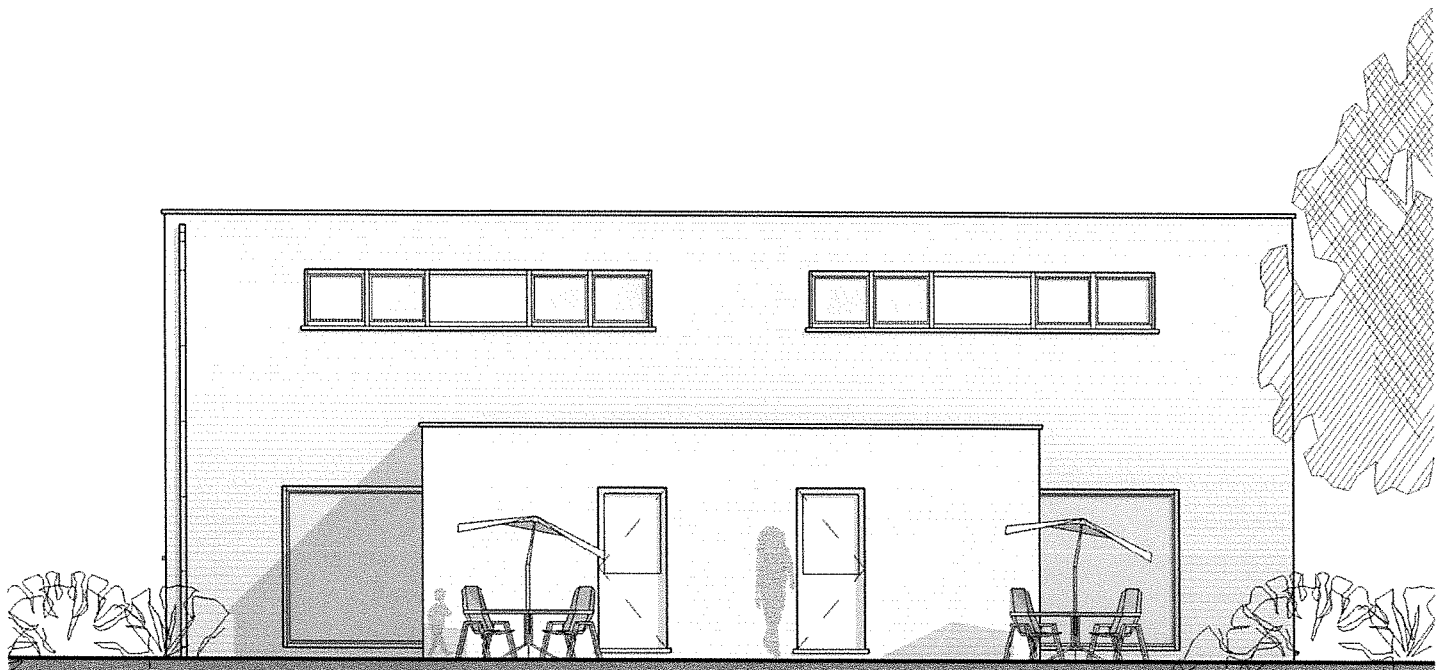
Achteraanzicht
