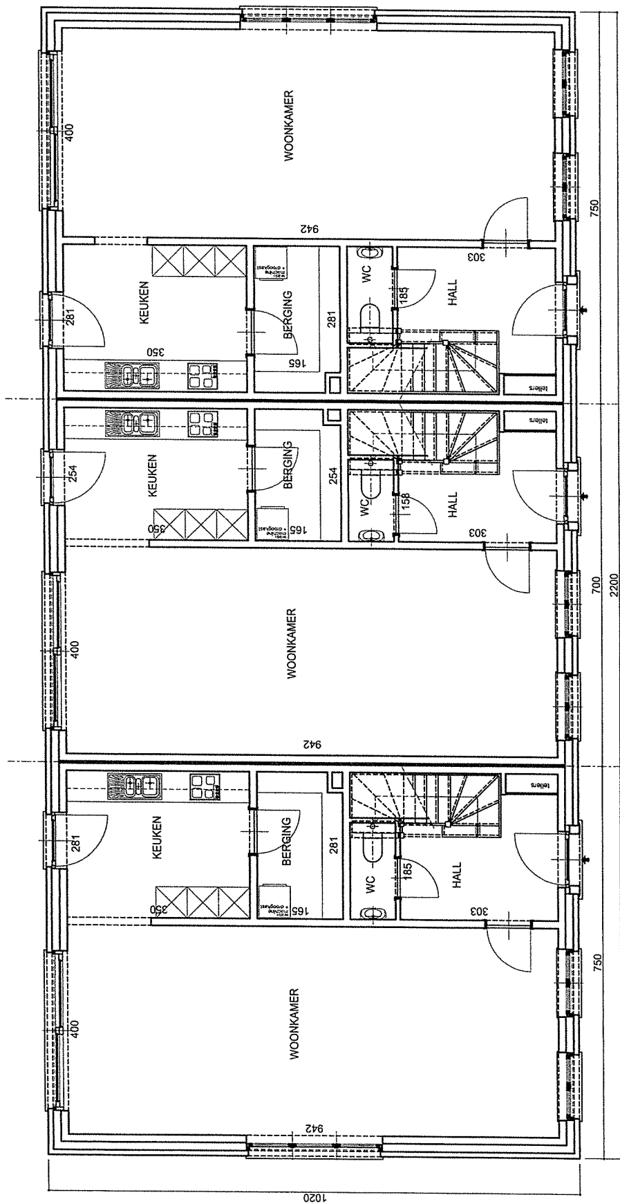
VOORONTWERP 1 GELIJKVLOERS
