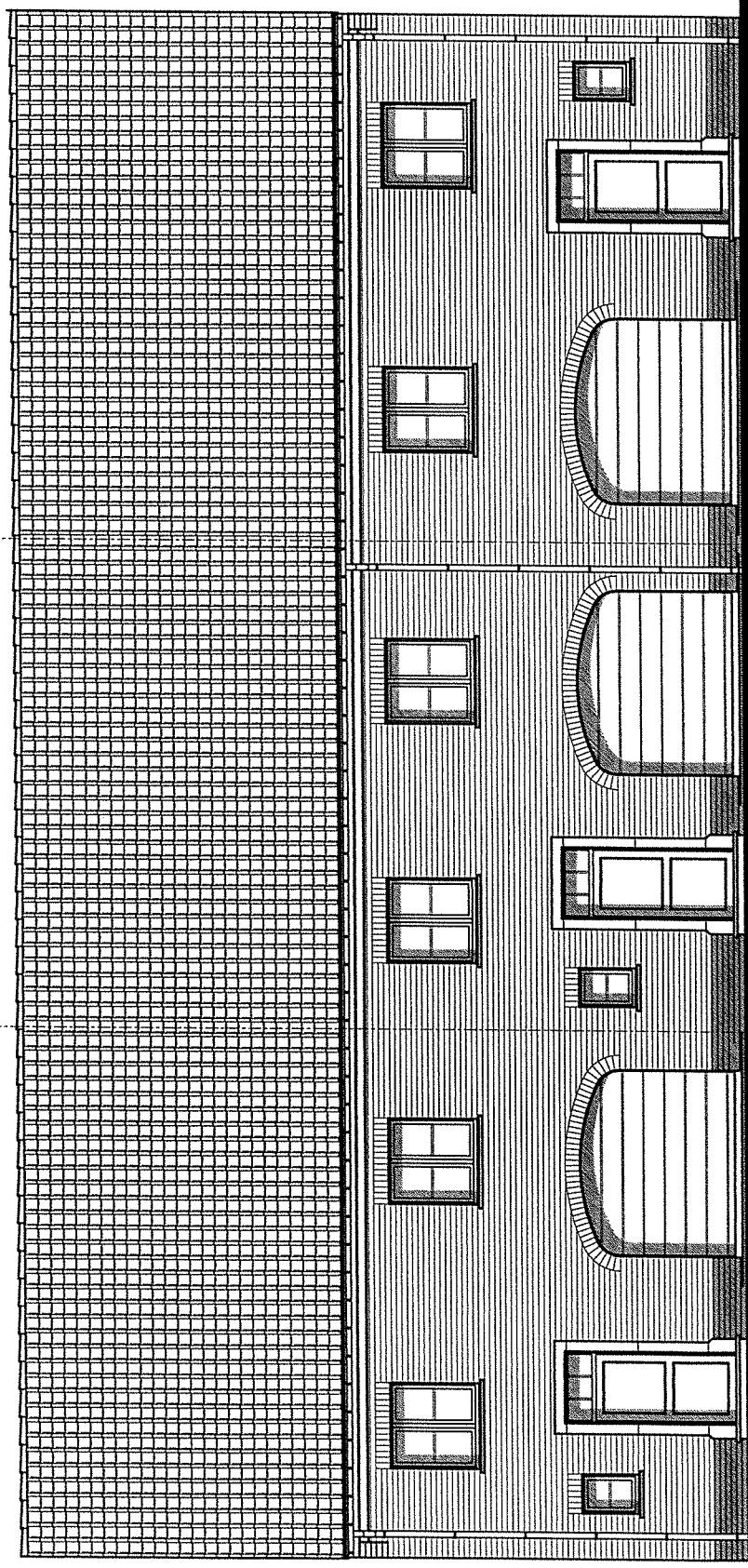
VOORONTWERP 2 VOORGEVEL
