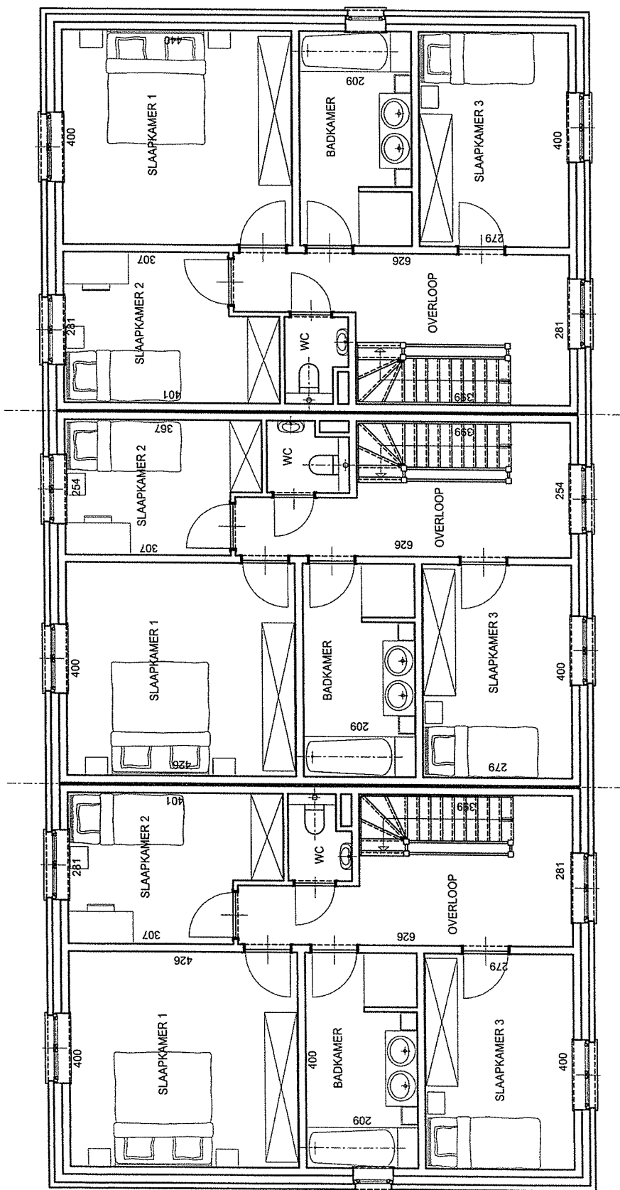
VOORONTWERP 1 VERDIEPING
