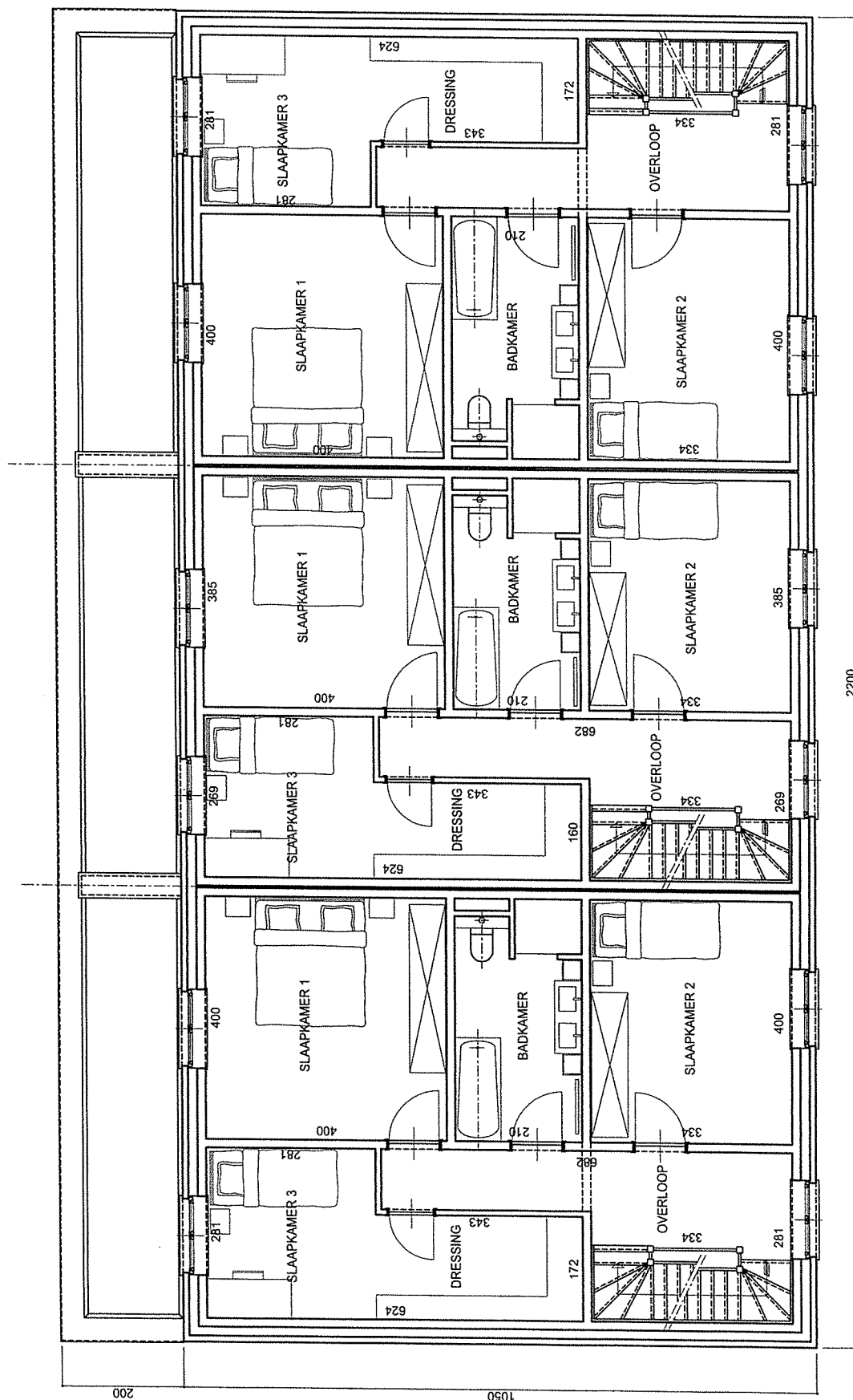
VOORONTWERP 2 VERDIEPING
