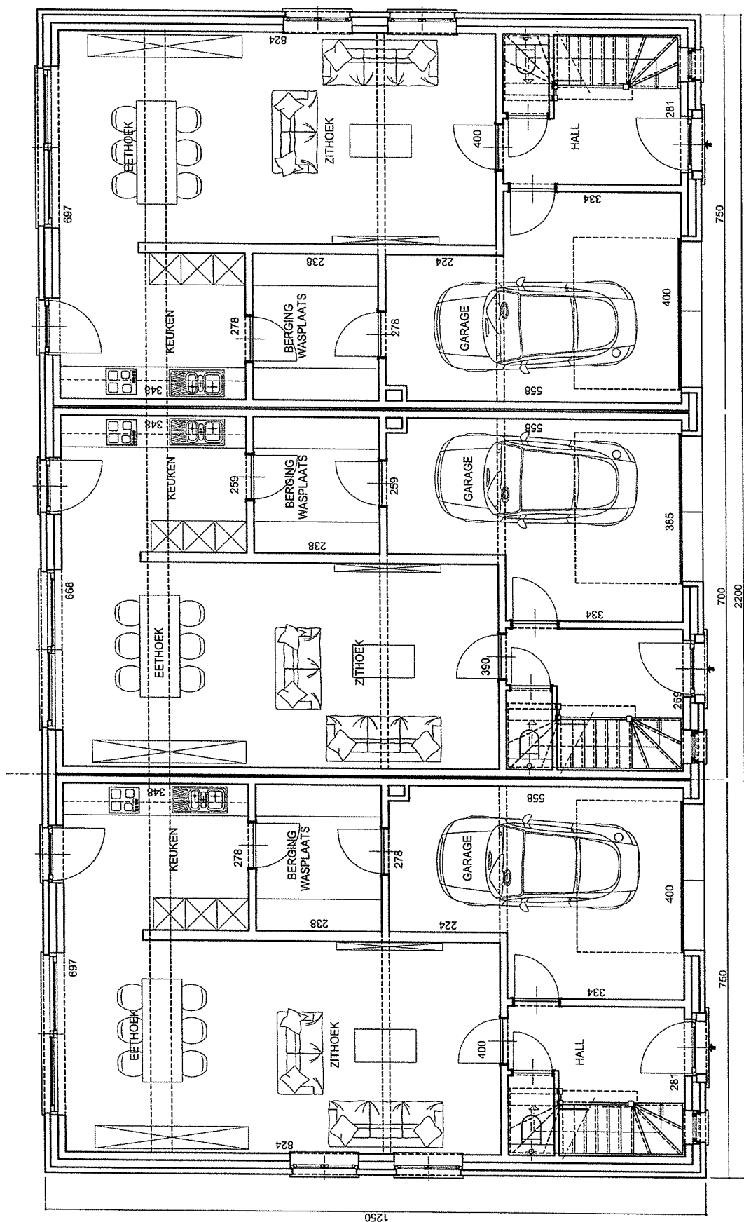
VOORONTWERP 2 GELIJKVLOERS
